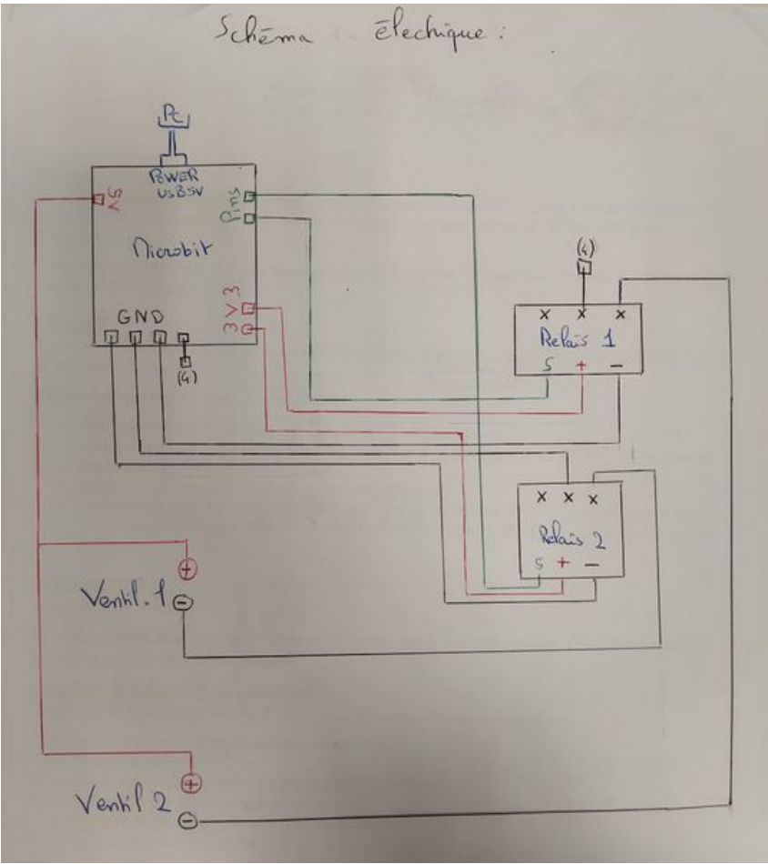
Taille de cet aperçu : 535 × 599 pixels. Fichier d'origine (3 352 × 3 754 pixels, taille du fichier : 2,27 Mio, type MIME : image/jpeg) Sauvez_ZIG_Schema_Cablage_1
