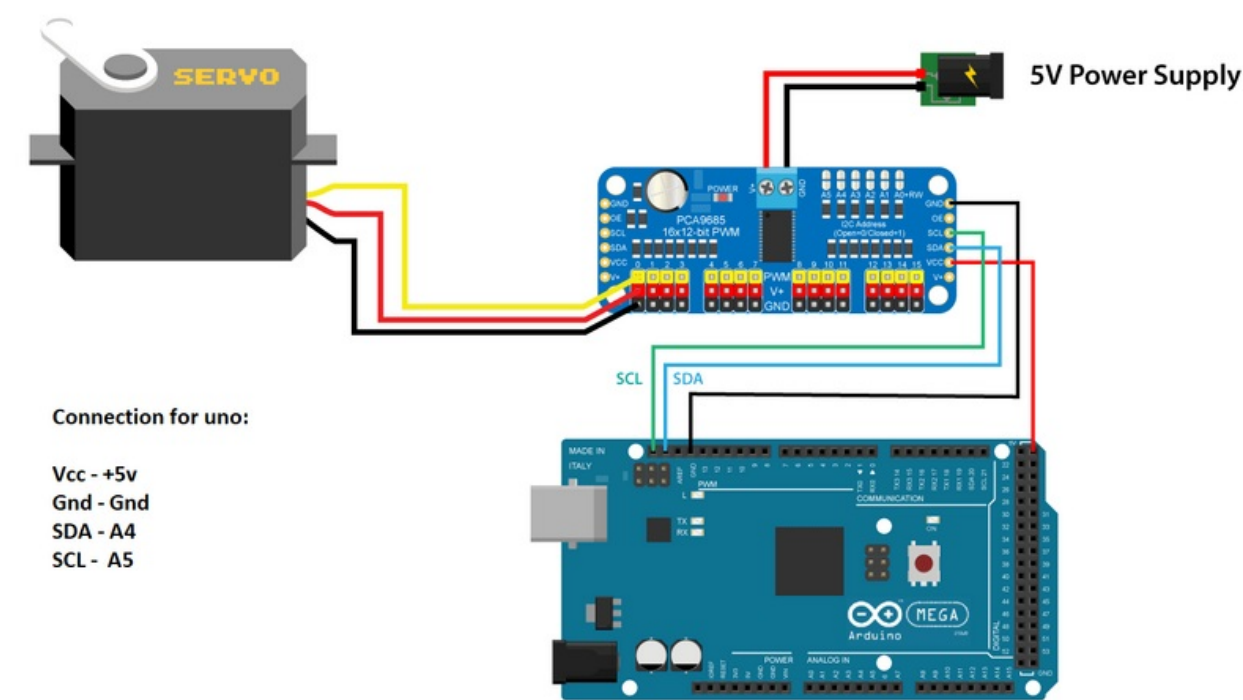
Taille de cet aperçu :800 × 466 pixels. Fichier d'origine (1 280 × 745 pixels, taille du fichier : 101 Kio, type MIME : image/png) Piano_automate_Arduino-and-PCA9685-Circuit-Schematic
