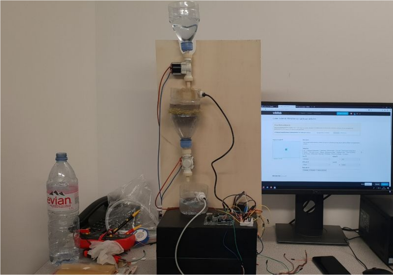
Taille de cet aperçu :800 × 559 pixels. Fichier d'origine (1 061 × 741 pixels, taille du fichier : 158 Kio, type MIME : image/jpeg) Filtration_sur_sable_par_arduino_20
