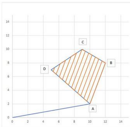
Grille de points pour un quadrilatère convexe fauché selon AB
